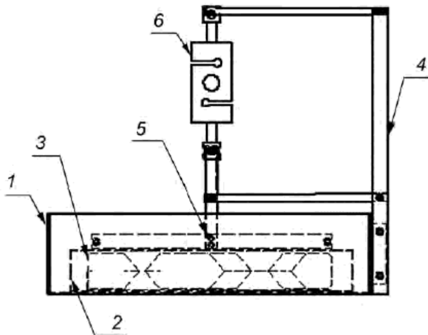
1 - емкость с водой; 2 - кассета; 3 - испытуемый образец; 4 - рама; 5 - фиксатор; 6 - динамометр Рисунок 2 - Испытательный стенд
